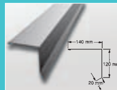
Gavelbeslag 1
