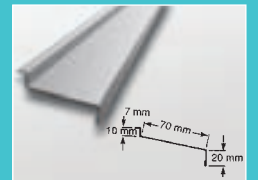
Fönsterbleck
