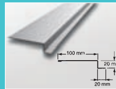
Foderbeslag
