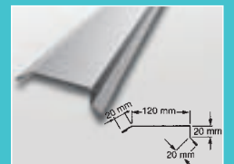
Vindskivebeslag
