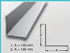
Innerhörn
