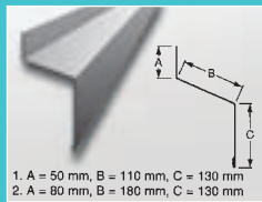
Droppbleck över skjutport
