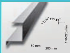
Gavelbeslag 2
