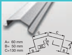
Ventilerad nock
