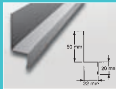
Sockelbeslag
