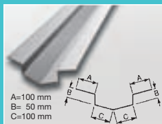
Försänkt rännadal
