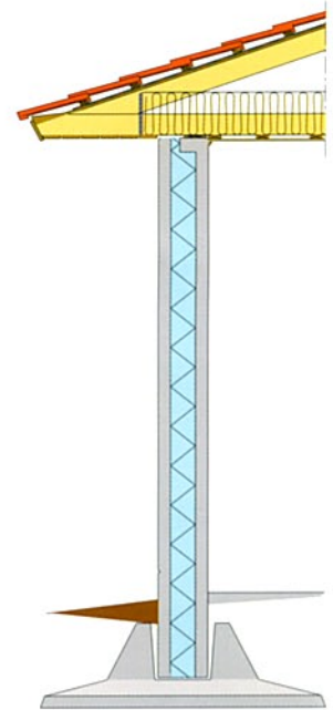
Fristående bärande väggelement i sandwichkonstruktion monterat i prefabricerad Finja holk.
