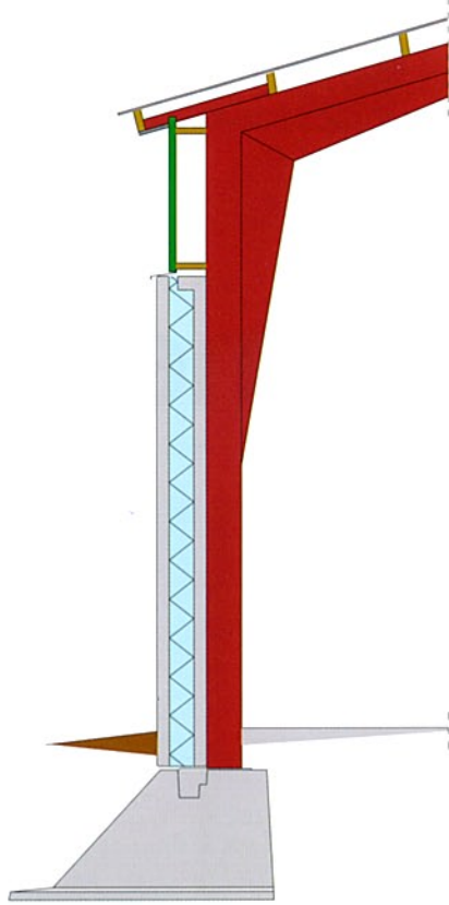
Väggelement i sandwichkonstruktion mot stål- eller betongstomme monterat på prefabricerad Finja plint.
