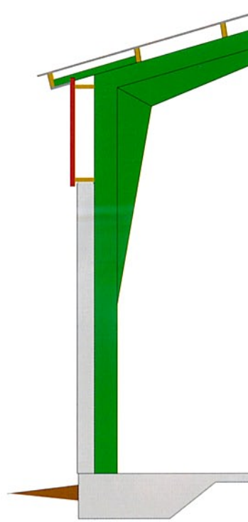
Homogent väggelement monterat mot stål- eller betongstomme på en kantförstyvad platta.
